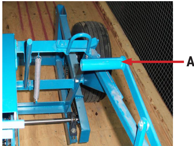
Fig.4 A - Levier de l'épandeur à gravier
